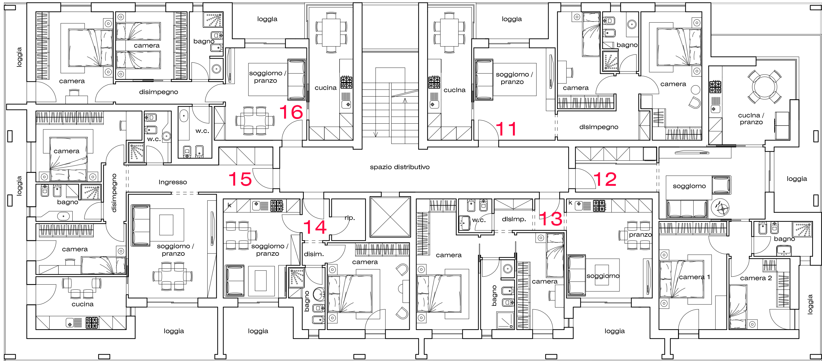
piano secondo scala 1/100
